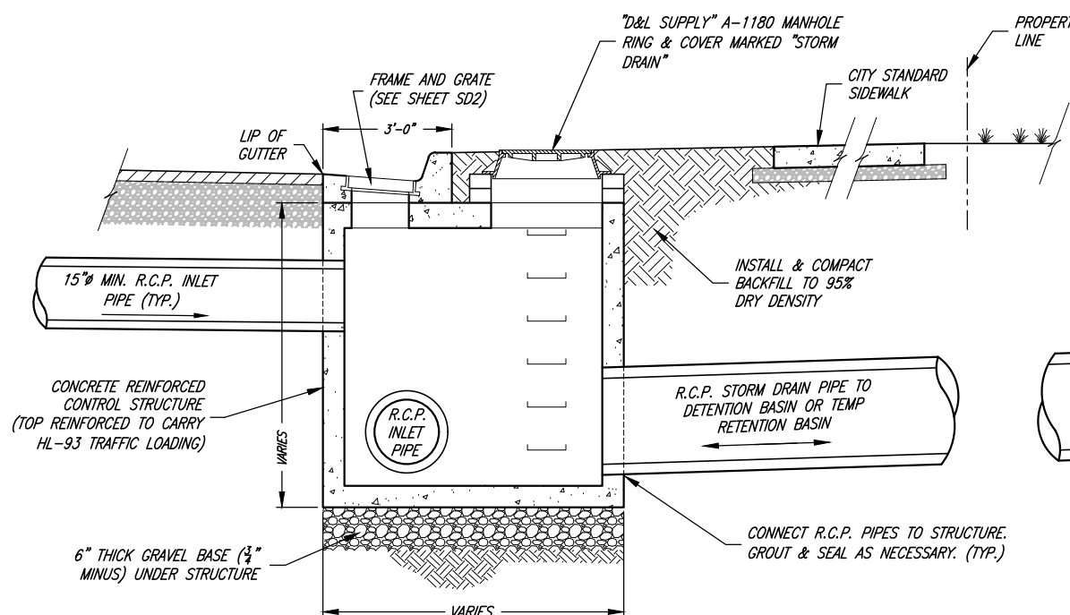
SECTION A-A
